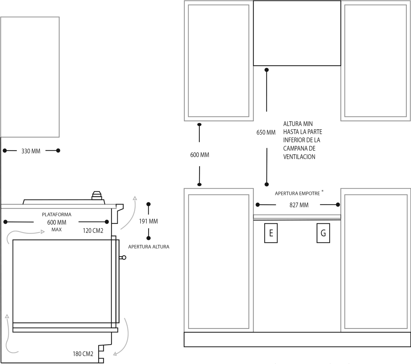
UBICACIÓN PARA CONEXIÓN ELÉCTRICA Y GAS Ancho de empotre * E *ubicación conexión eléctrica G *ubicación conexión gas VISTA FRONTAL
